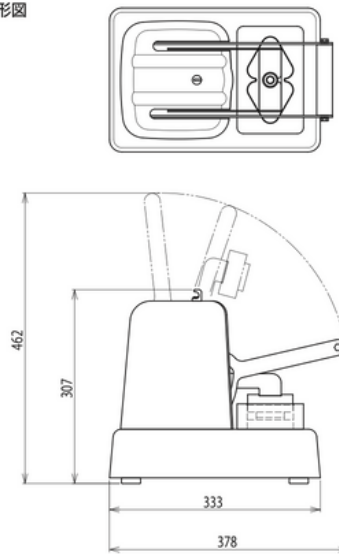
■外形図
